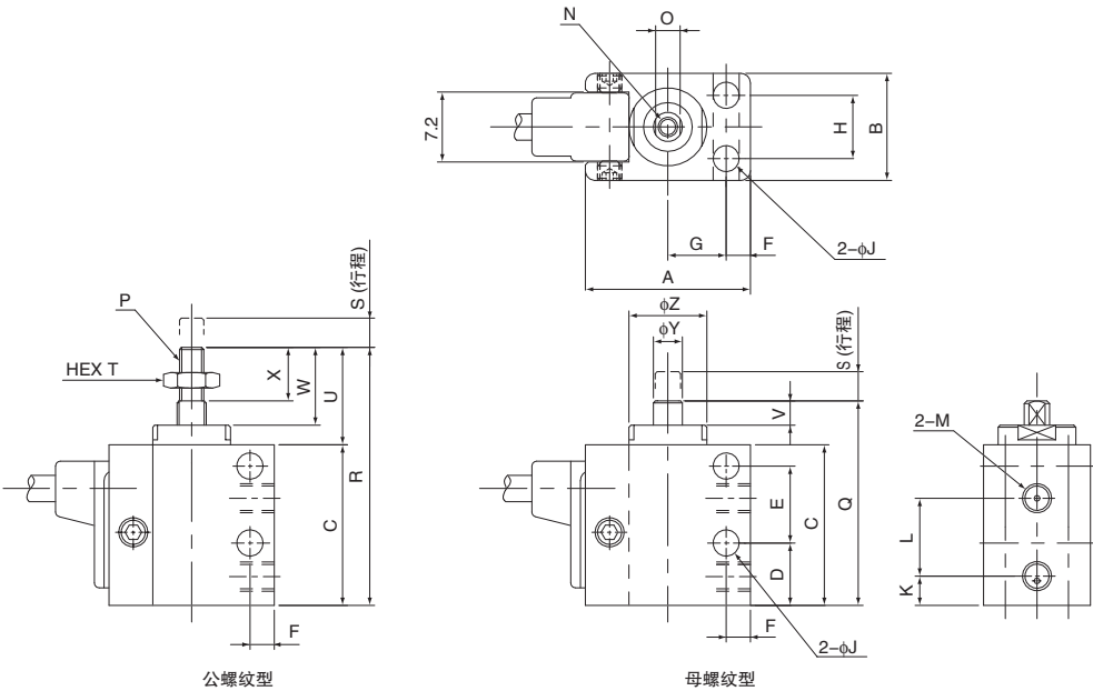
外形尺寸图
