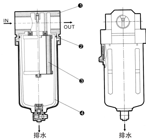
构造图
