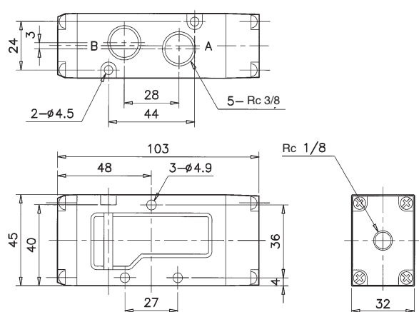
单先导阀 CMV310
