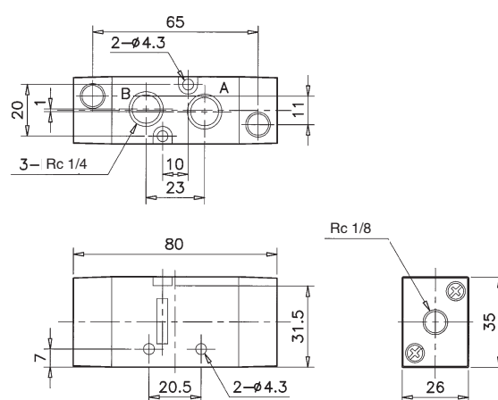
双先导阀 CMV220
