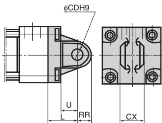
单耳环型
