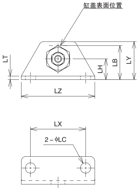
脚座型 LB
