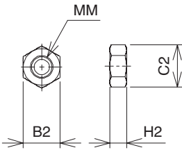
活塞杆前端螺母
