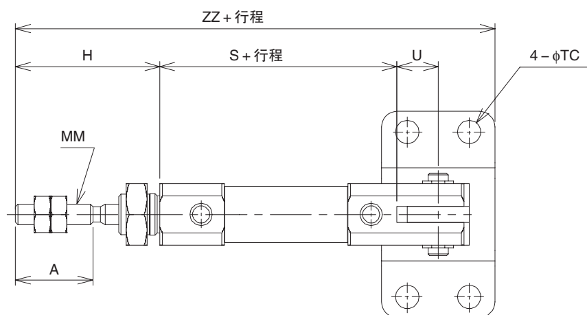
轴销型 \phi 10 \sim \phi 16 T
