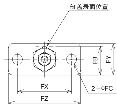
法兰型 FA
