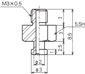
TN-PS-2A-M3
