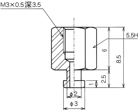
TN-PS-2A-M3F
