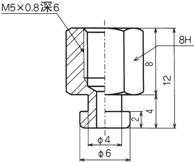
TN-PS-10-M5F
