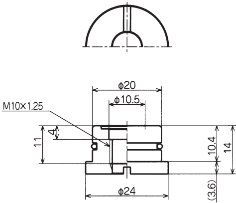
TN-PH-65-M10
